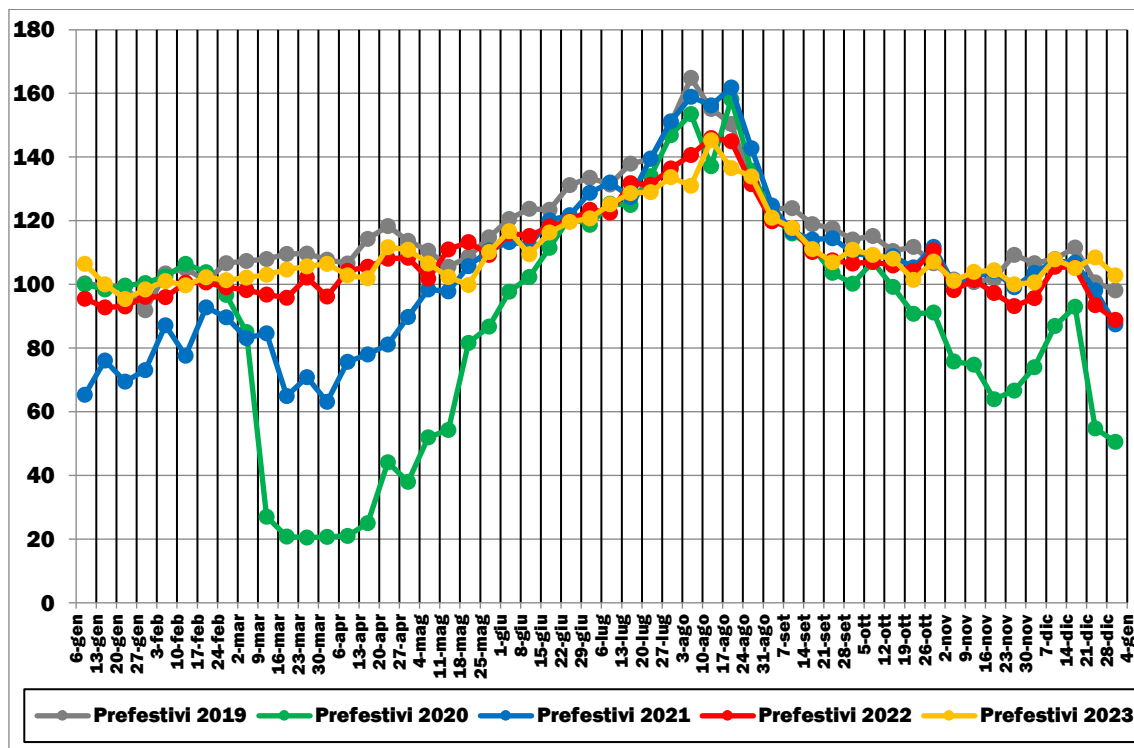
FIGURA 2.5: TRAFFICI STRADALI GIORNALIERI MEDI (LEGGERI + PESANTI) NEI GIORNI PREFESTIVI (GENNAIO 2019-DICEMBRE 2023)
