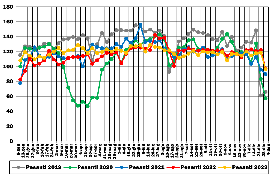
FIGURA 2.28: TRAFFICI STRADALI GIORNALIERI MEDI PESANTI (GENNAIO 2019-DICEMBRE 2023)
