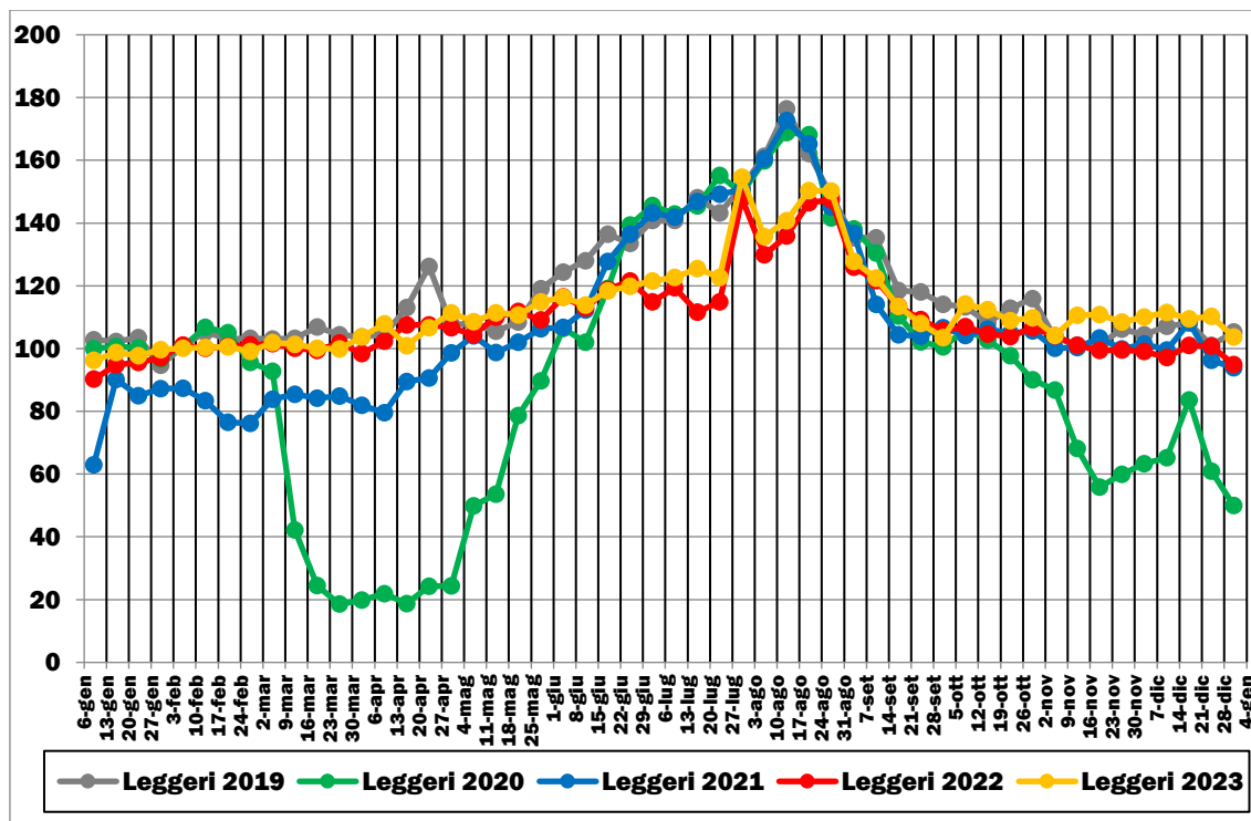
FIGURA 2.29: TRAFFICI STRADALI GIORNALIERI MEDI LEGGERI (GENNAIO 2019-DICEMBRE 2023)
