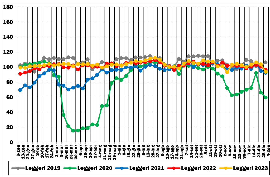
FIGURA 2.17: TRAFFICI STRADALI GIORNALIERI MEDI LEGGERI (GENNAIO 2019-DICEMBRE 2023)
