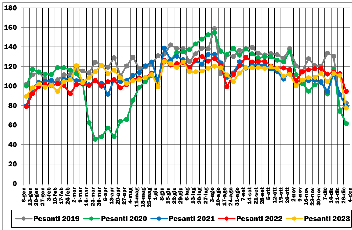
FIGURA 2.36: TRAFFICI STRADALI GIORNALIERI MEDI PESANTI (GENNAIO 2019-DICEMBRE 2023)
