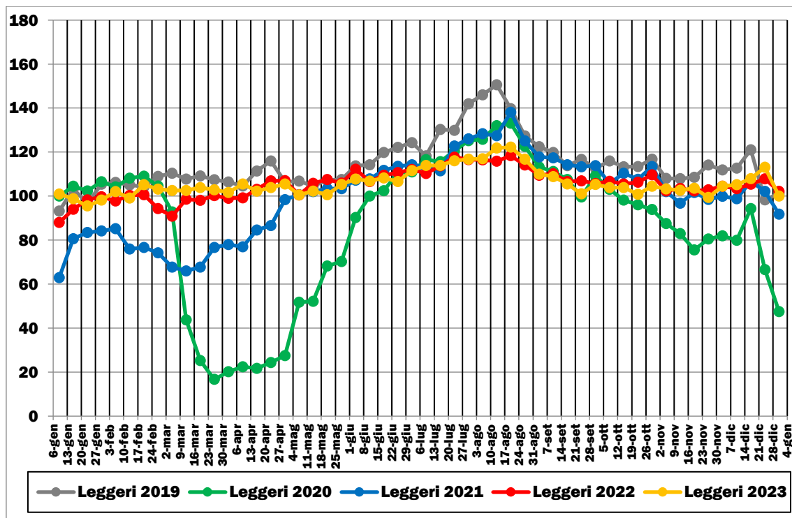
FIGURA 2.41: TRAFFICI STRADALI GIORNALIERI MEDI LEGGERI (GENNAIO 2019-DICEMBRE 2023)
