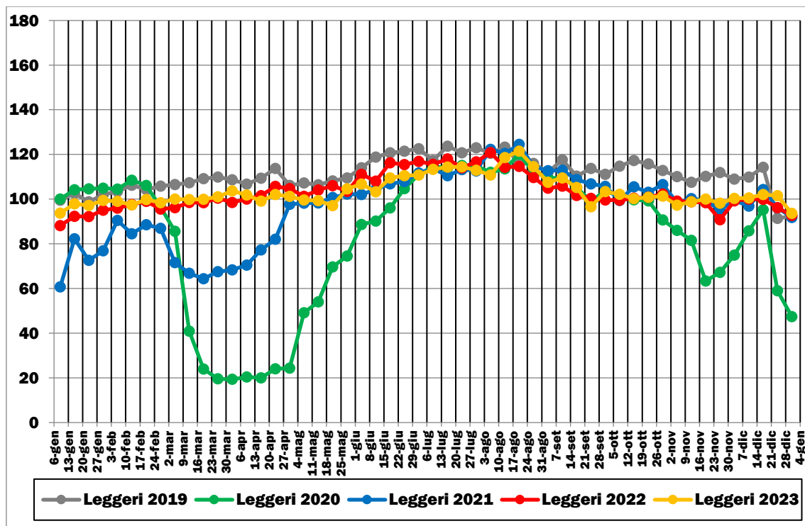
FIGURA 2.27: TRAFFICI STRADALI GIORNALIERI MEDI LEGGERI (GENNAIO 2019-DICEMBRE 2023)
