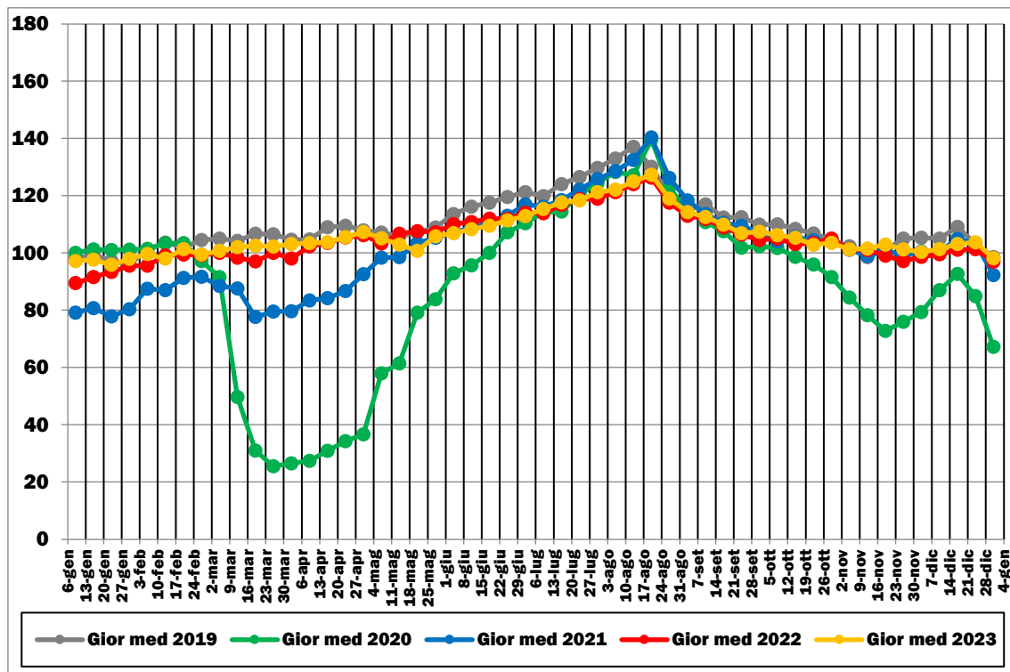
FIGURA 2.6: TRAFFICI STRADALI GIORNALIERI MEDI (LEGGERI + PESANTI) NEL GIORNO MEDIO (GENNAIO 2019-DICEMBRE 2023)
