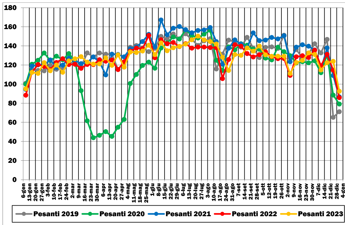
FIGURA 2.34: TRAFFICI STRADALI GIORNALIERI MEDI PESANTI (GENNAIO 2019-DICEMBRE 2023)
