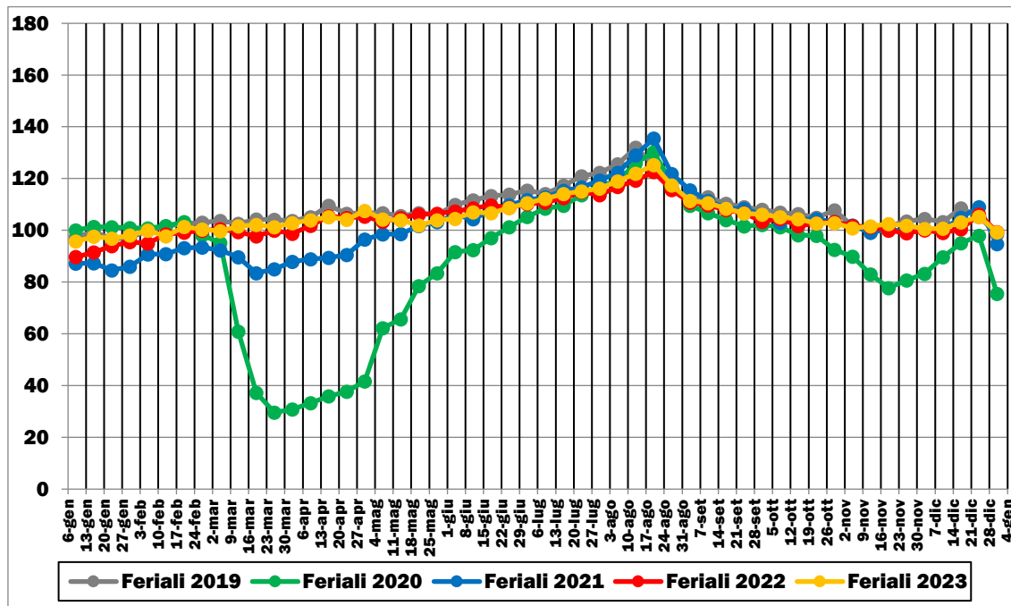
FIGURA 2.3: TRAFFICI STRADALI GIORNALIERI MEDI (LEGGERI + PESANTI) NEI GIORNI FERIALI (GENNAIO 2019-DICEMBRE 2023)
