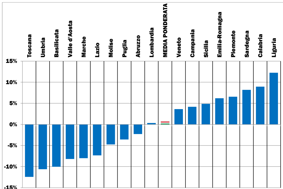
FIGURA 2.11: VARIAZIONE % DEI TRAFFICI STRADALI GIORNALIERI MEDI PESANTI NEL IV TRIMESTRE 2023 RISPETTO AD ANALOGO PERIODO PRE-COVID-19
