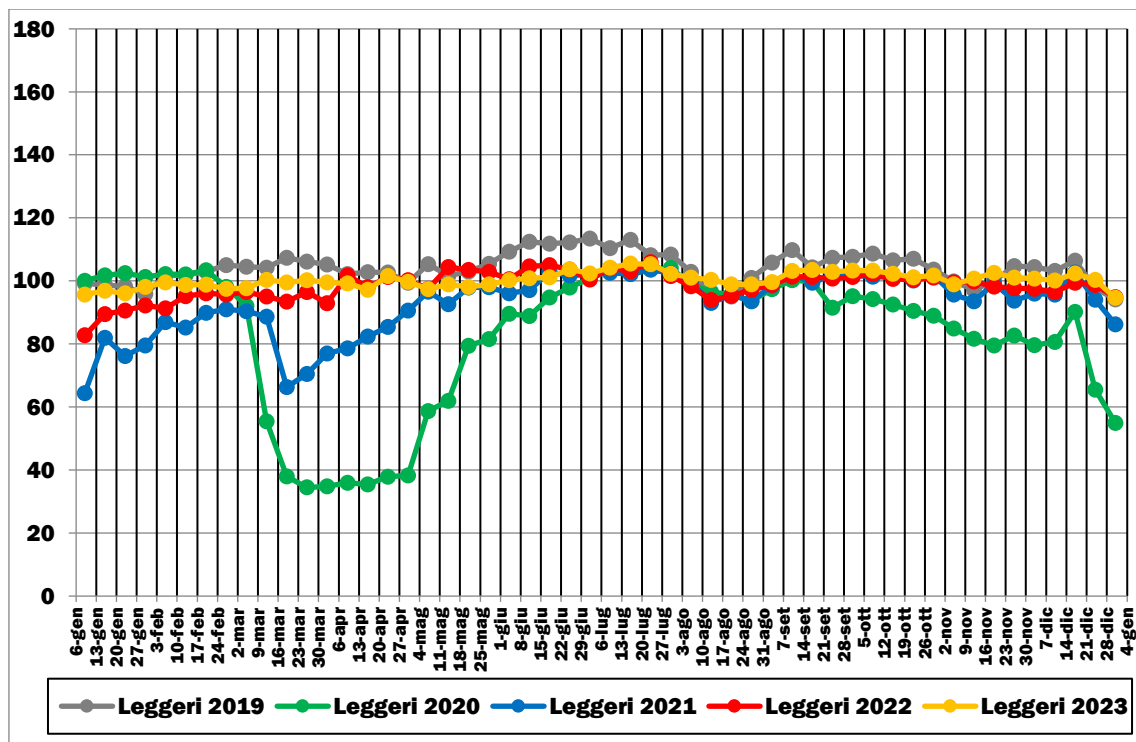
FIGURA 2.25: TRAFFICI STRADALI GIORNALIERI MEDI LEGGERI (GENNAIO 2019-DICEMBRE 2023)
