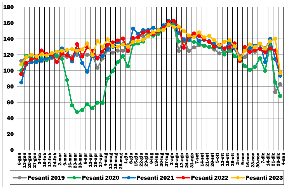
FIGURA 2.38: TRAFFICI STRADALI GIORNALIERI MEDI PESANTI (GENNAIO 2019-DICEMBRE 2023)
