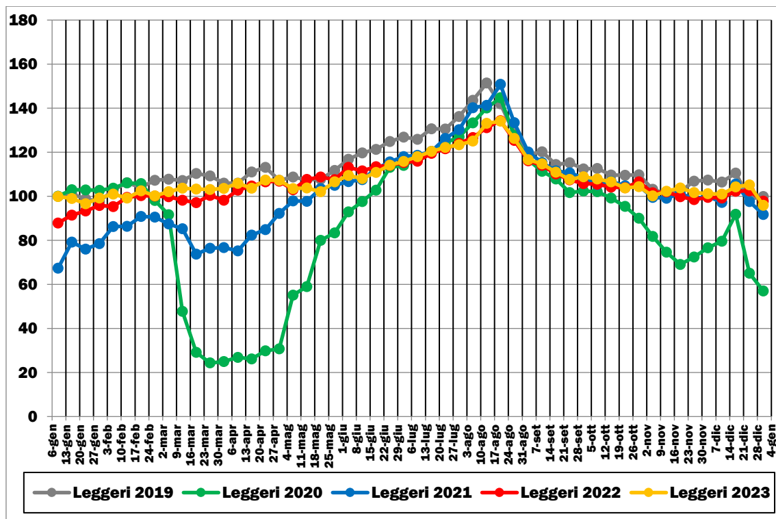
FIGURA 2.7: TRAFFICI STRADALI GIORNALIERI MEDI LEGGERI (GENNAIO 2019-DICEMBRE 2023)
