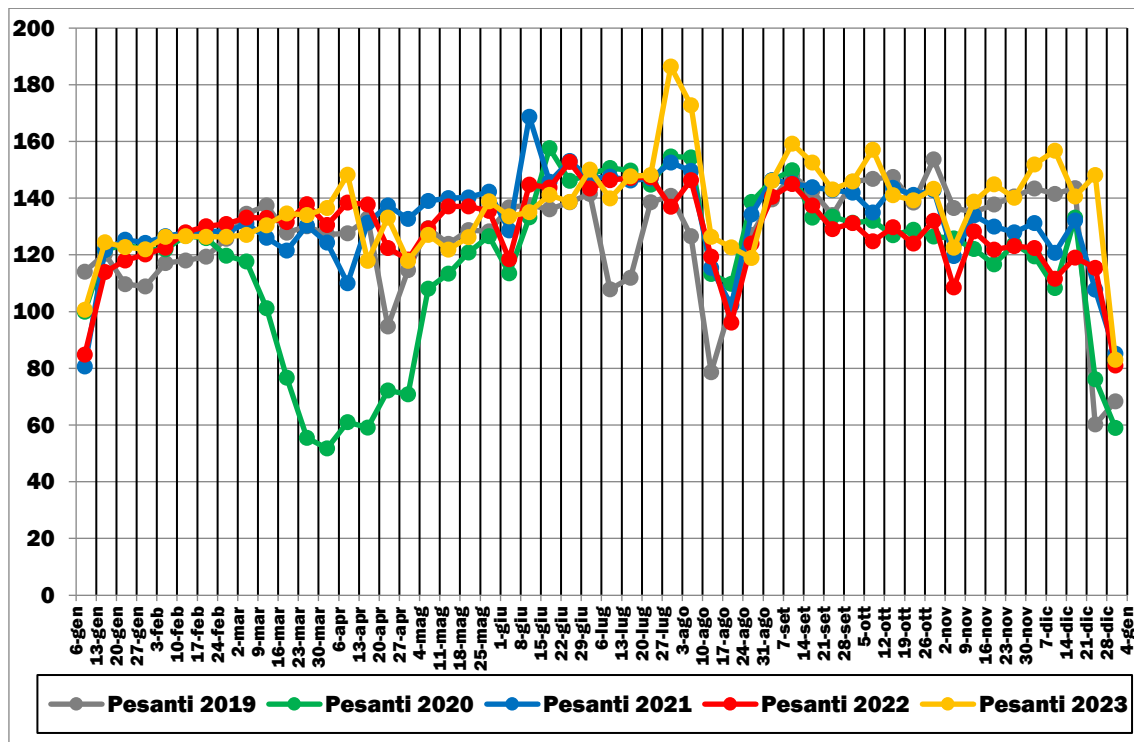
FIGURA 2.14: TRAFFICI STRADALI GIORNALIERI MEDI PESANTI (GENNAIO 2019-DICEMBRE 2023)
