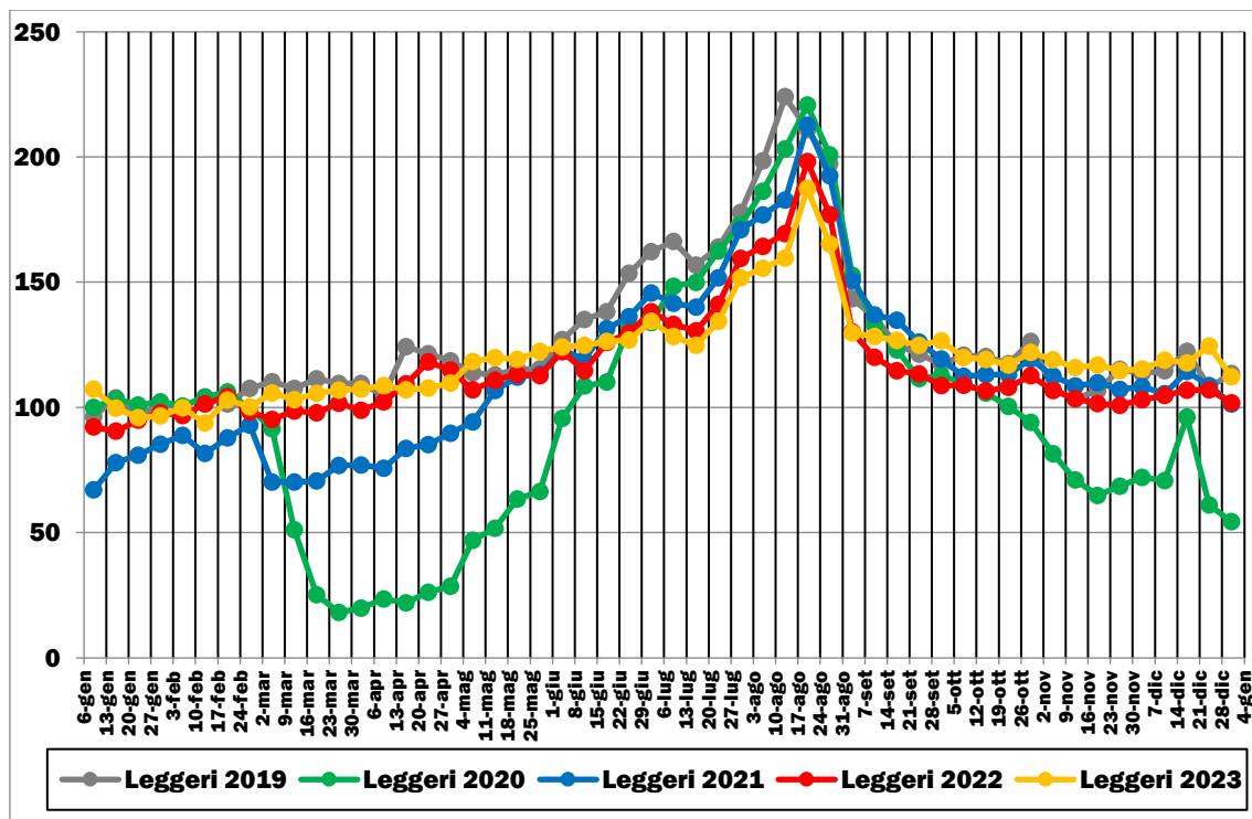
FIGURA 2.35: TRAFFICI STRADALI GIORNALIERI MEDI LEGGERI (GENNAIO 2019-DICEMBRE 2023)
