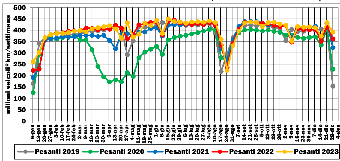
FIGURA 2.2: TRAFFICI AUTOSTRADALI DI VEICOLI*KM PESANTI (GENNAIO 2019-DICEMBRE 2023)
