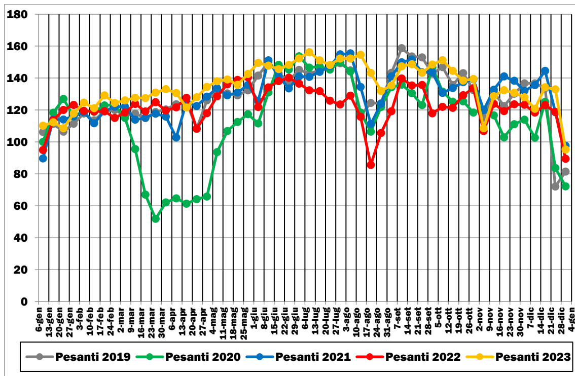
FIGURA 2.40: TRAFFICI STRADALI GIORNALIERI MEDI PESANTI (GENNAIO 2019-DICEMBRE 2023)
