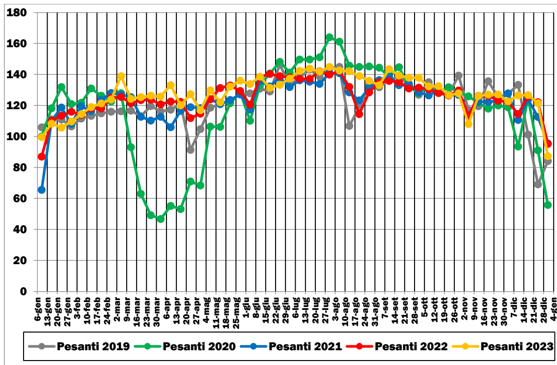
FIGURA 2.24: TRAFFICI STRADALI GIORNALIERI MEDI PESANTI (GENNAIO 2019-DICEMBRE 2023)
