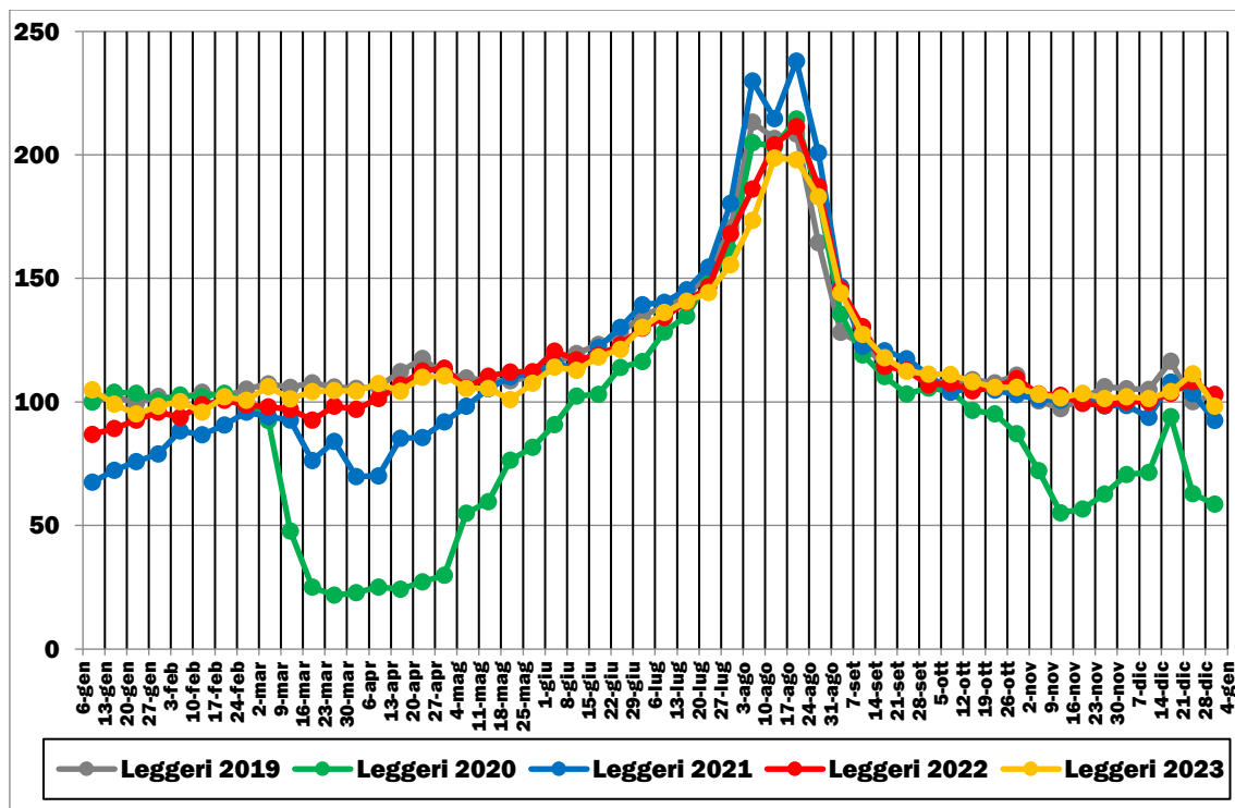
FIGURA 2.37: TRAFFICI STRADALI GIORNALIERI MEDI LEGGERI (GENNAIO 2019-DICEMBRE 2023)
