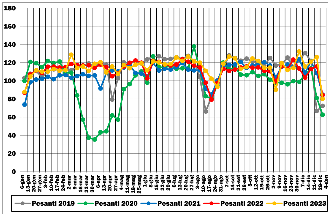
FIGURA 2.18: TRAFFICI STRADALI GIORNALIERI MEDI PESANTI (GENNAIO 2019-DICEMBRE 2023)
