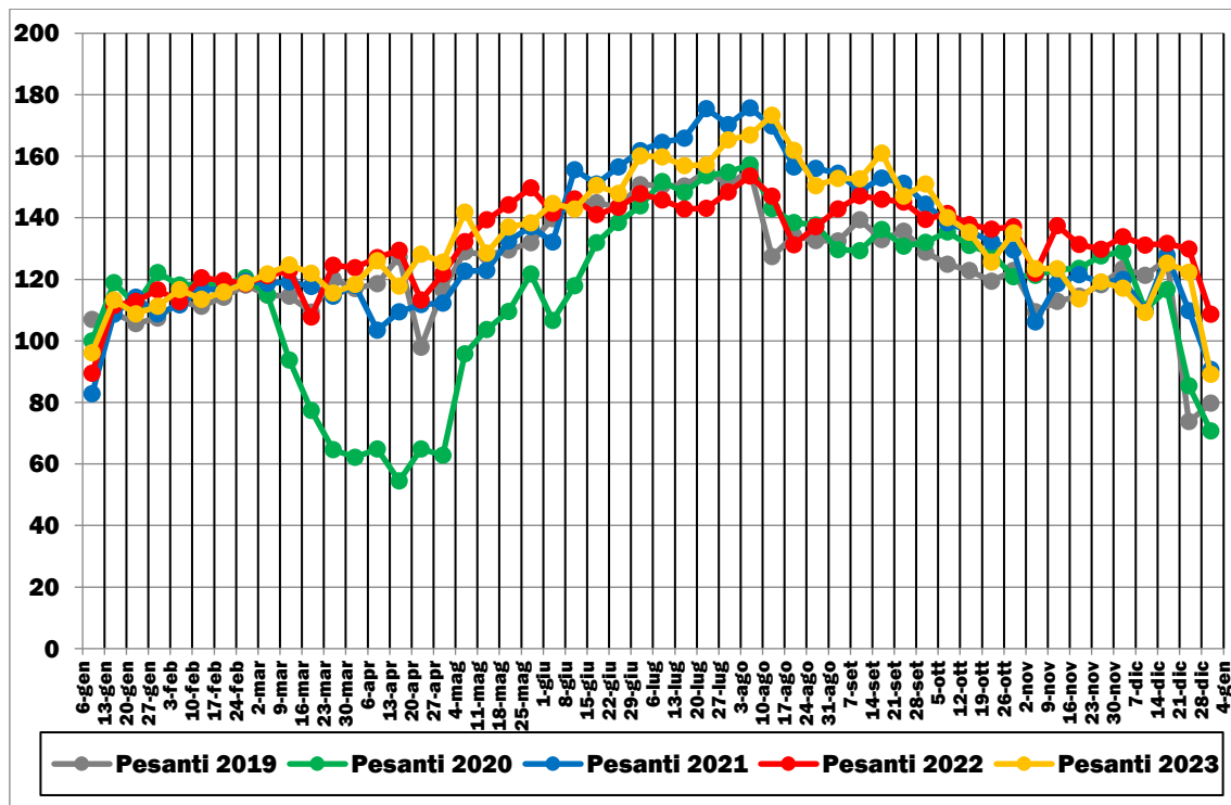
FIGURA 2.46: TRAFFICI STRADALI GIORNALIERI MEDI PESANTI (GENNAIO 2019-DICEMBRE 2023)
