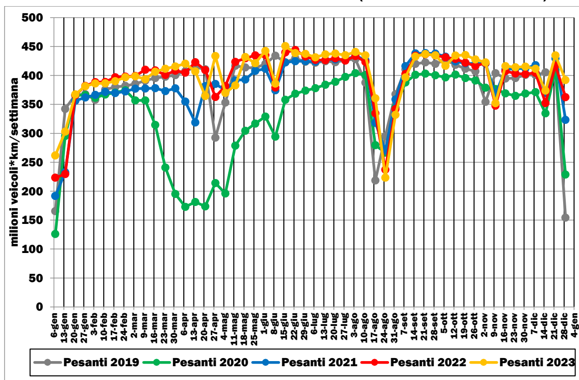
FIGURA E.5: TRAFFICI AUTOSTRADALI DI VEICOLI*KM PESANTI (GENNAIO 2019-DICEMBRE 2023)
