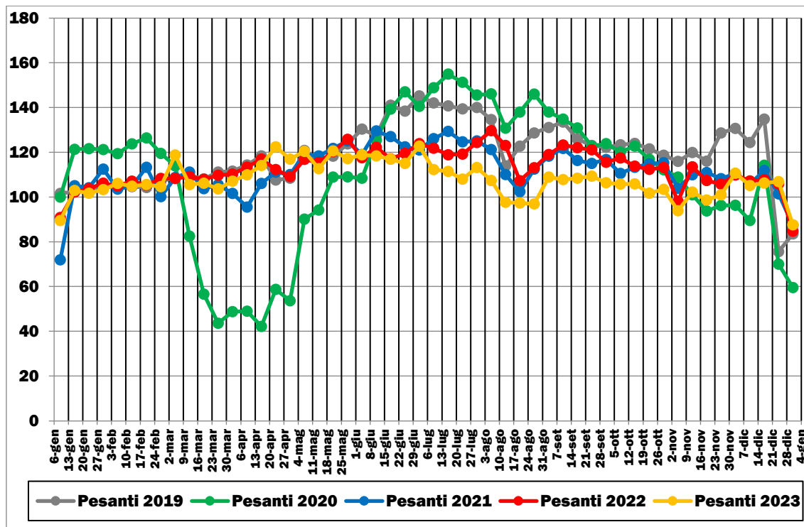
FIGURA 2.30: TRAFFICI STRADALI GIORNALIERI MEDI PESANTI (GENNAIO 2019-DICEMBRE 2023)
