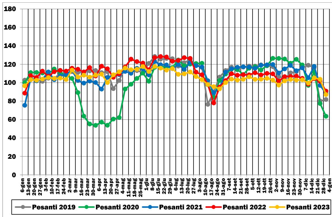
FIGURA 2.26: TRAFFICI STRADALI GIORNALIERI MEDI PESANTI (GENNAIO 2019-DICEMBRE 2023)
