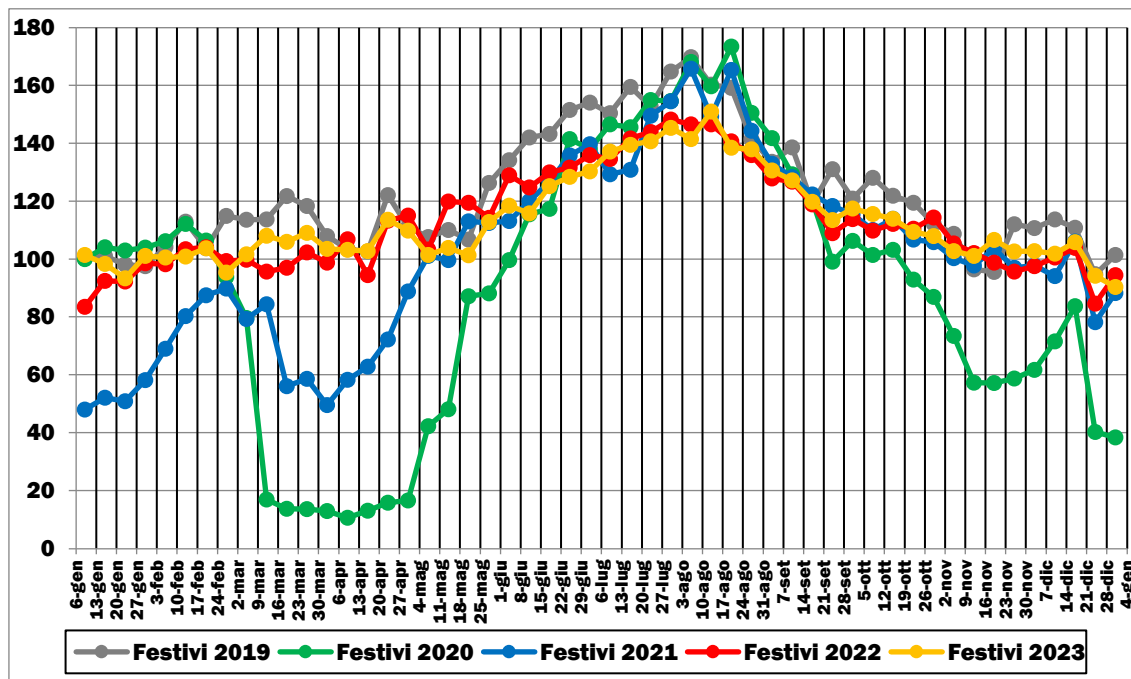
FIGURA 2.4: TRAFFICI STRADALI GIORNALIERI MEDI (LEGGERI + PESANTI) NEI GIORNI FESTIVI (GENNAIO 2019-DICEMBRE 2023)
