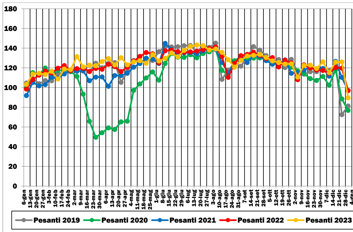
FIGURA 2.48: TRAFFICI STRADALI GIORNALIERI MEDI PESANTI (GENNAIO 2019-DICEMBRE 2023)
