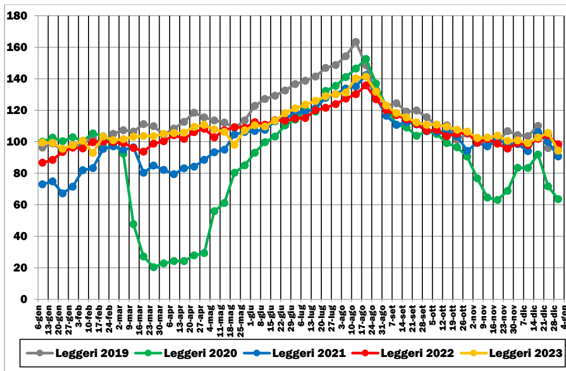
FIGURA 2.47: TRAFFICI STRADALI GIORNALIERI MEDI LEGGERI (GENNAIO 2019-DICEMBRE 2023)
