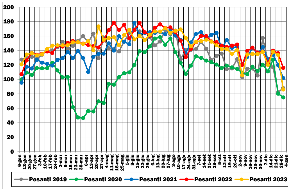
FIGURA 2.16: TRAFFICI STRADALI GIORNALIERI MEDI PESANTI (GENNAIO 2019-DICEMBRE 2023)
