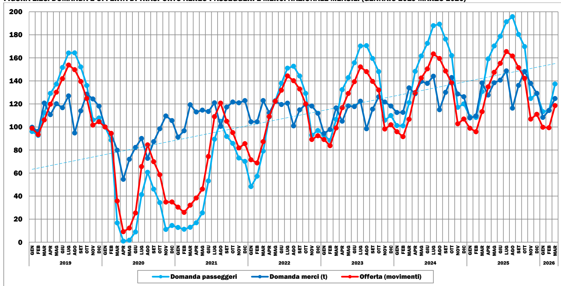
FIGURA E.23: DOMANDA E OFFERTA DI TRASPORTO AEREO PASSEGGERI E MERCI NAZIONALE MENSILI (GENNAIO 2019-MARZO 2026)
