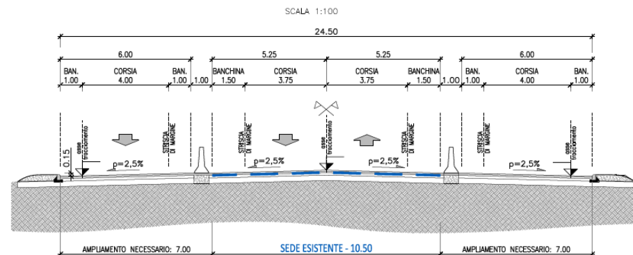
SEZIONE TIPO MINIMA NECESSARIA ("C1" EXTRAURBANA SECONDARIA CON STRADE DI SERVIZIO)
