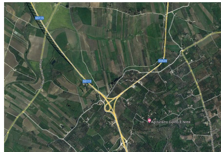
FIGURA 2-16- SS 115 Svincoli di collegamento con la SS624
