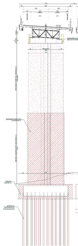
Figura 3-12 – Sezione trasversale e interventi di rinforzo impalcato asse principale
