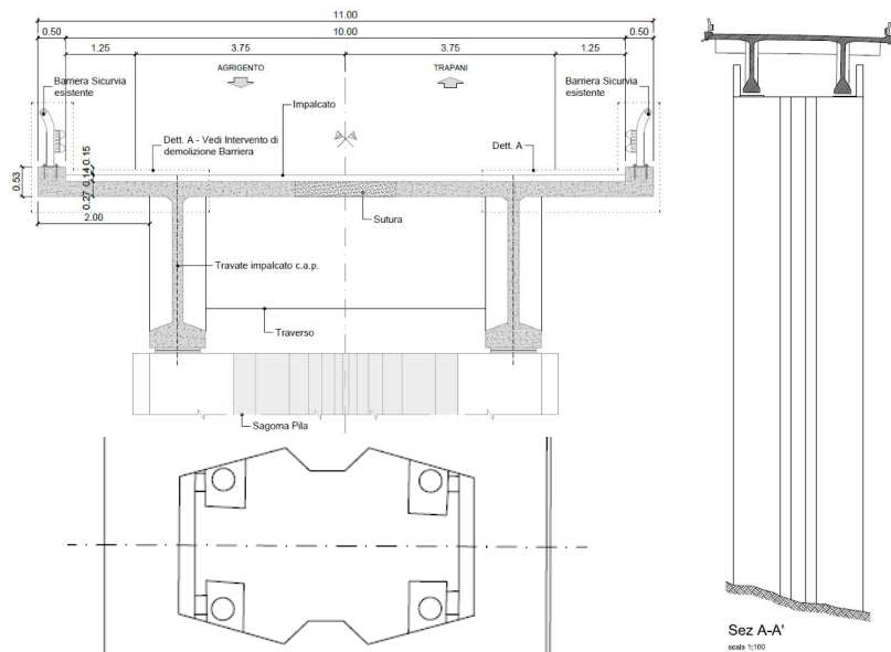
Figura 3-11 – Sezione trasversale impalcato e pile esistenti asse principale - Alternative 2A e 2B
