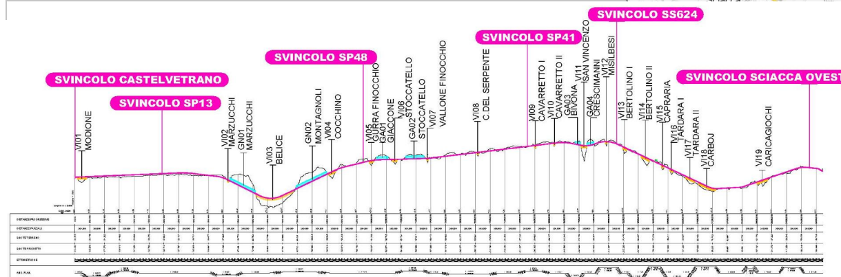
Figura 3-8 - Planimetria e profilo di progetto - Alternativa 1
