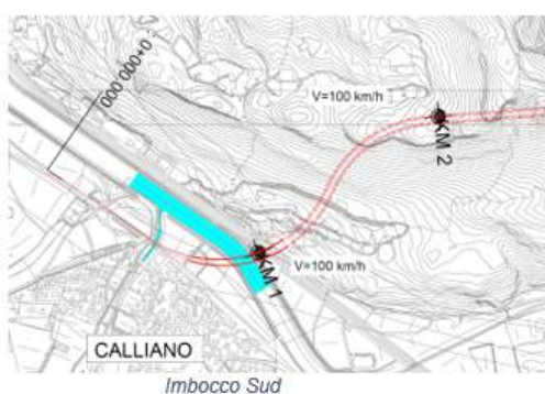
Stralcio studio condotto da ITALFERR per la soluzione in Destra Adige
