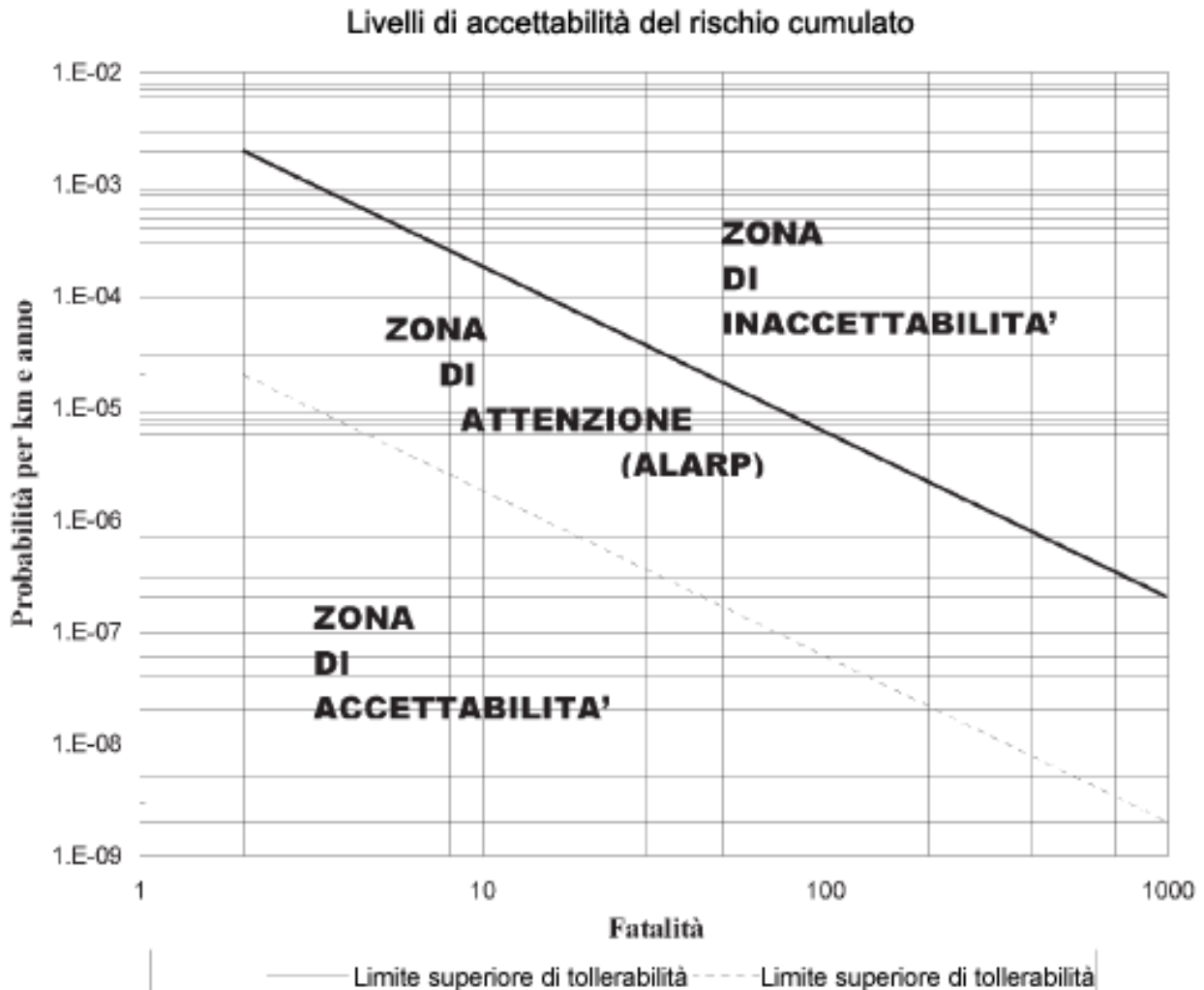
Tavola 4.3.I: Obiettivi di sicurezza: livelli di accettabilità del Rischio Cumulato nelle gallerie ferroviarie.
