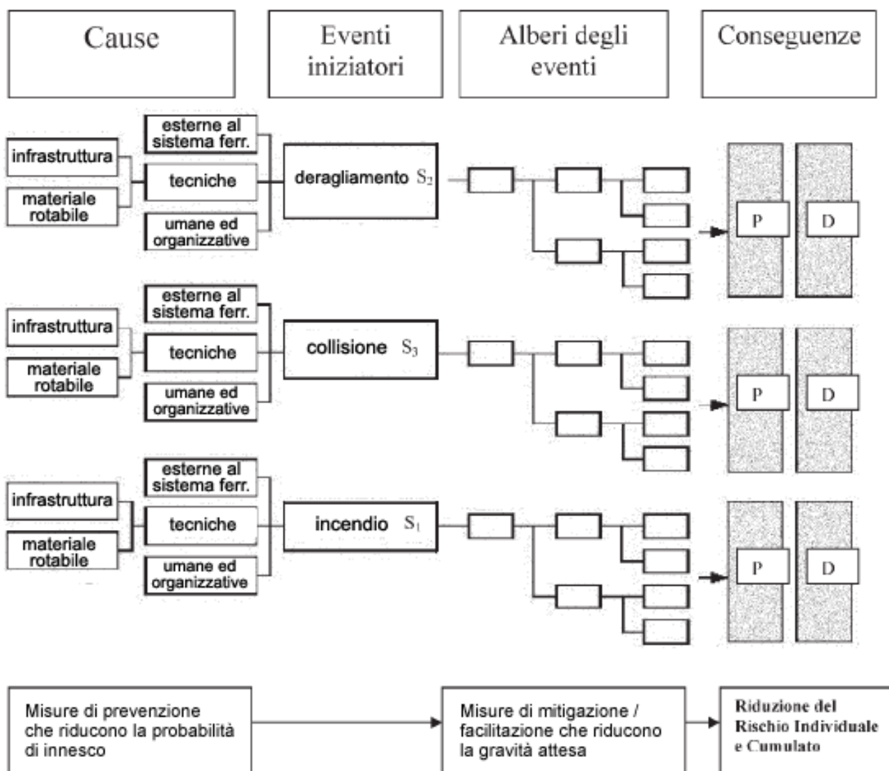
Tavola 3.4.I: Schema della procedura estesa
